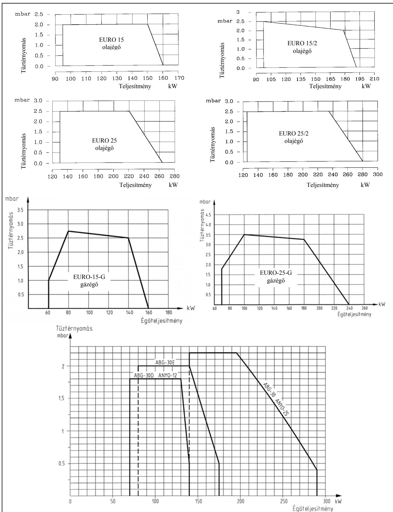
9. ábra Kommunális gáz- és olajégők tűztérnyomás-teljesítmény jelleggörbéi
