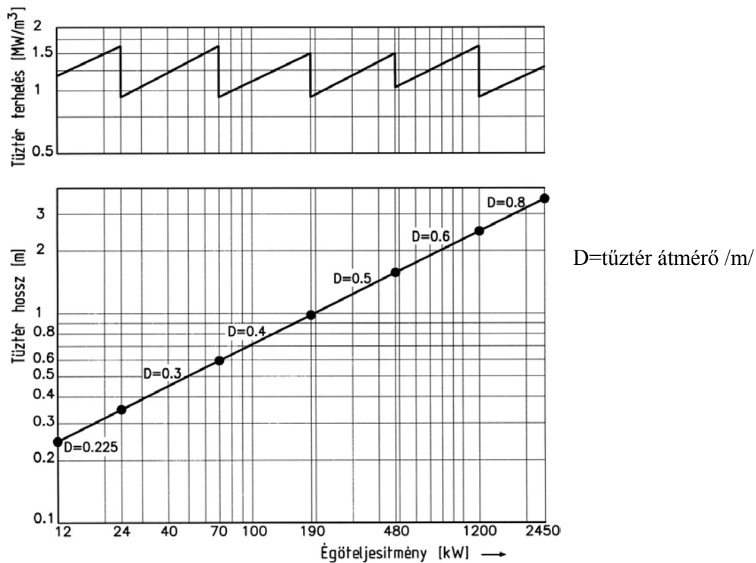
5. ábra Tüztér méretek EN 676 szerint
