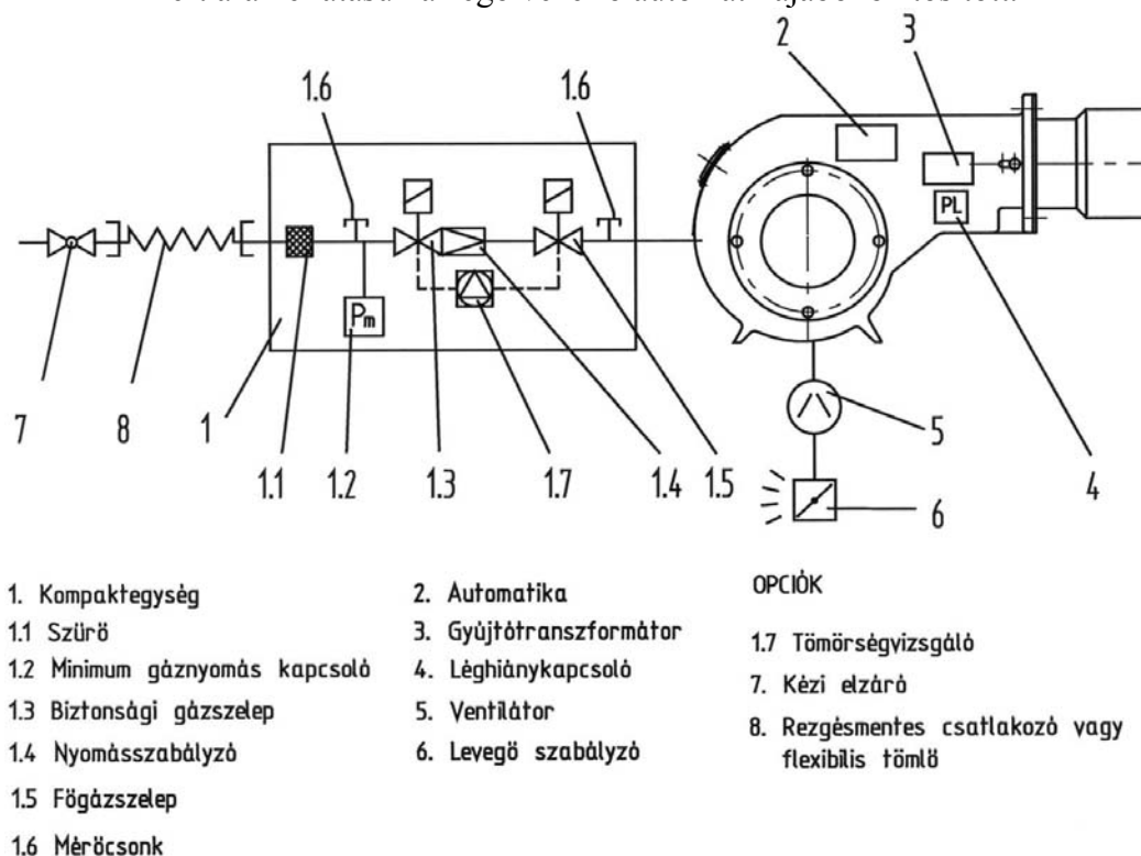
14. ábra Kétpont szabályzás elvi kapcsolási rajza
